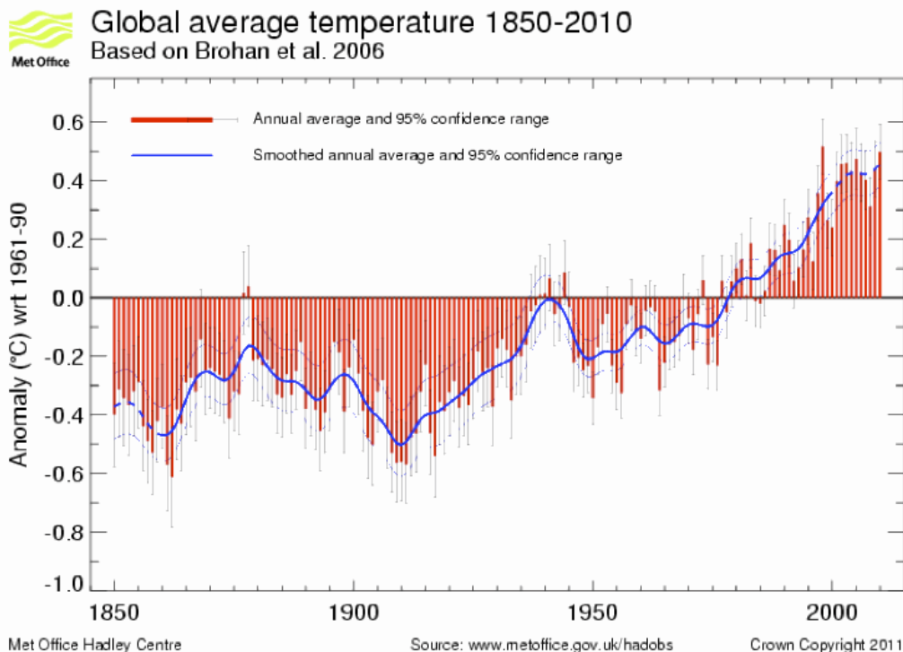
Abbildung 1 Die blaue mittlere Trendlinie zeigt globale Mitteltemperatur wie sie vom britischen Met-Office [0] von 1850 bis Ende 2010 im Internet
