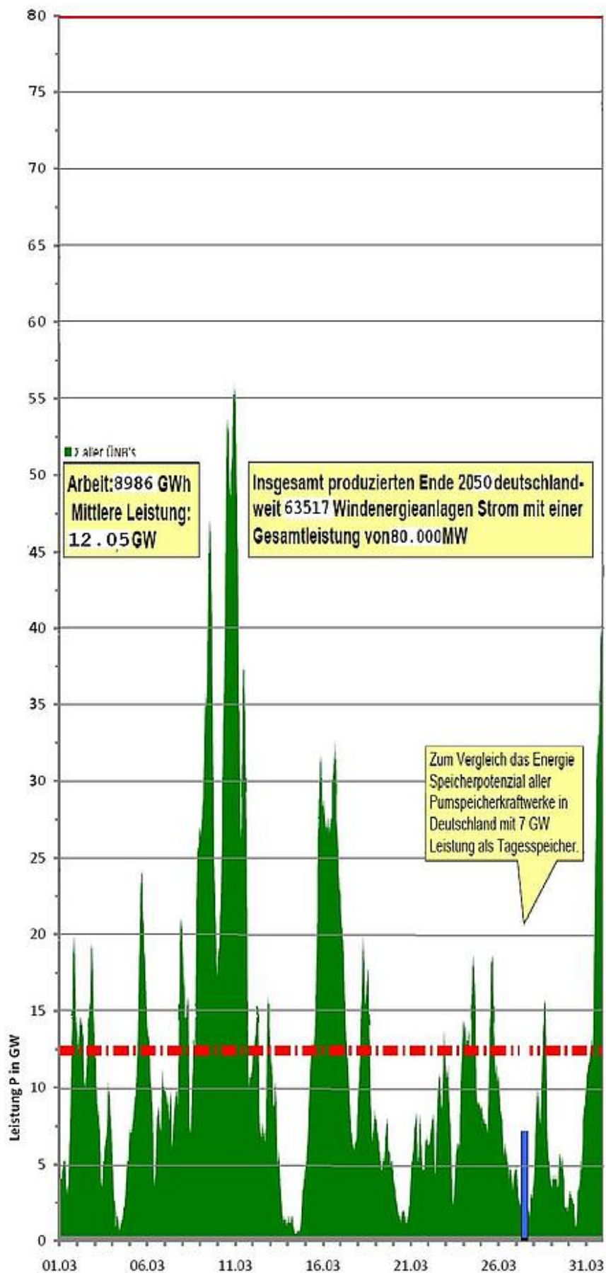
Ganglinie der zeitgleichen Windleistungseinspeisung vom 1.3.2050 bis zum 31.3.2050 als 1/4 h Messwerte
