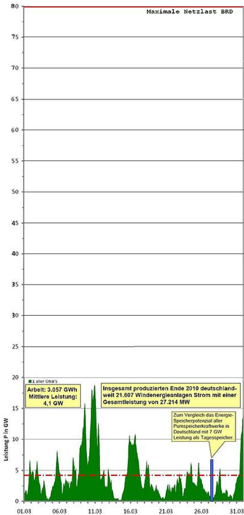
Ganglinie der zeitgleichen Windleistungseinspeisung vom 1.3.2011 bis zum 31.3.2011 als 1/4 h Messwerte
