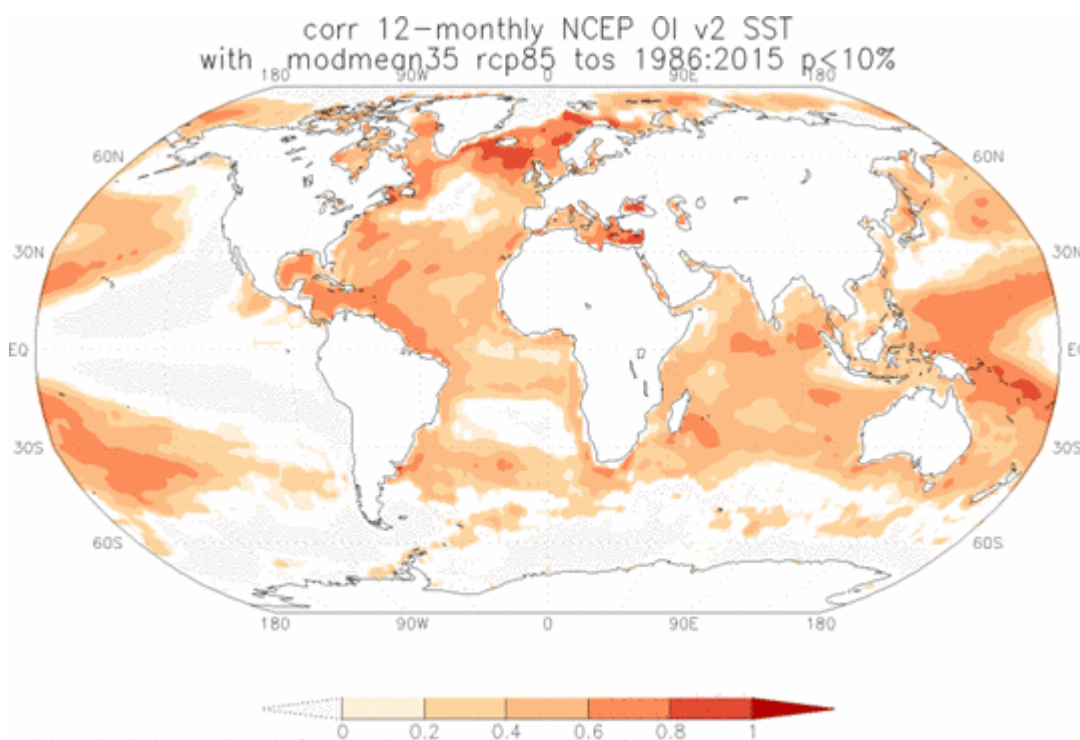
Abb.2: Die Korrelation (Grad der Übereinstimmung) zwischen dem Modellmittel und den Beobachtungen für die Ozeane, hergestellt mit dem „Climate Explorer“. 0=sehr schlechte Korrelation, 1=sehr gute Korrelation.
