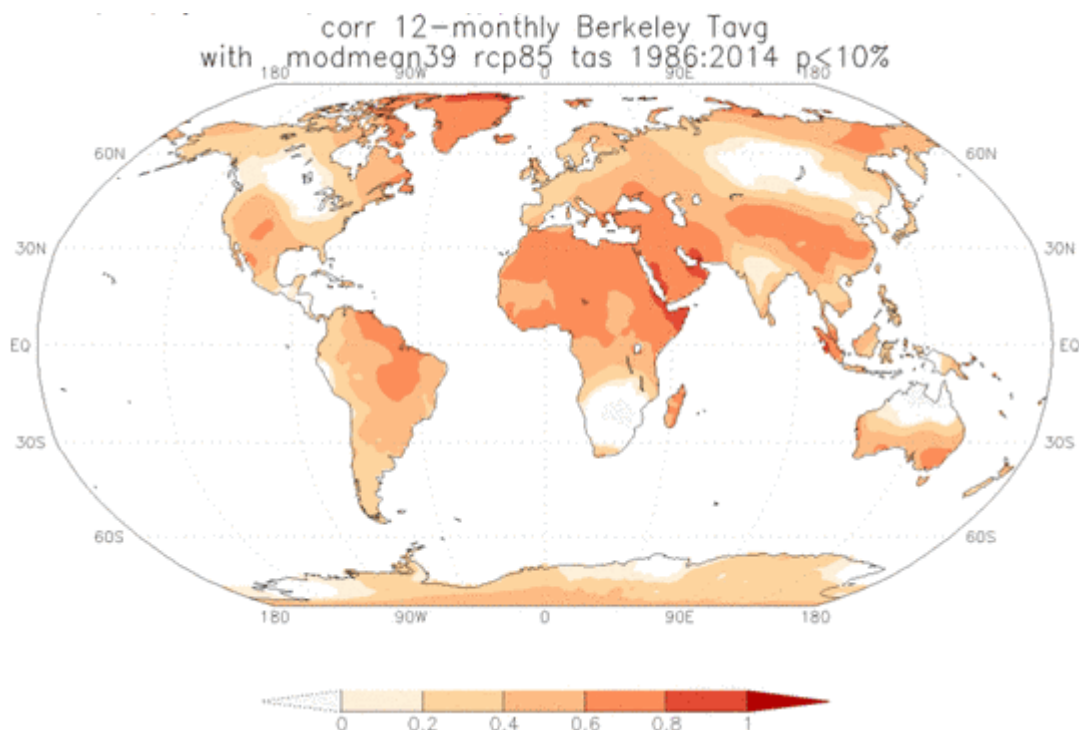
Abb.1: Korrelation (Grad der Übereinstimmung) zwischen Modellen und realer Temperaturentwicklung für Landflächen. Das Bild wurde hergestellt mit dem „Climate Explorer“. 0=sehr schlechte Korrelation, 1=sehr gute Korrelation.
