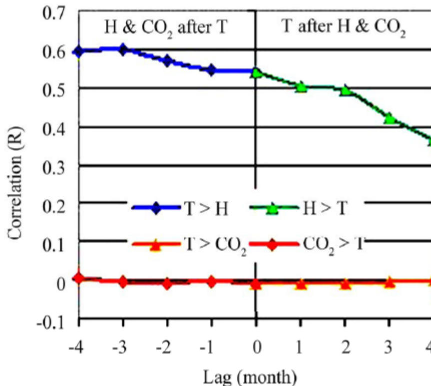
Abb. 22. Ursache und Wirkung der spezifischen Luftfeuchte in der Atmosphäre in Verbindung mit Temperaturveränderungen: Korrelation auf monatlicher Skala im Vergleich zur CO2-Korrelation zwischen 1983 und 2003. Temperatur des tropischen Bandes; CO2 von Mauna Loa (CDIAC)
