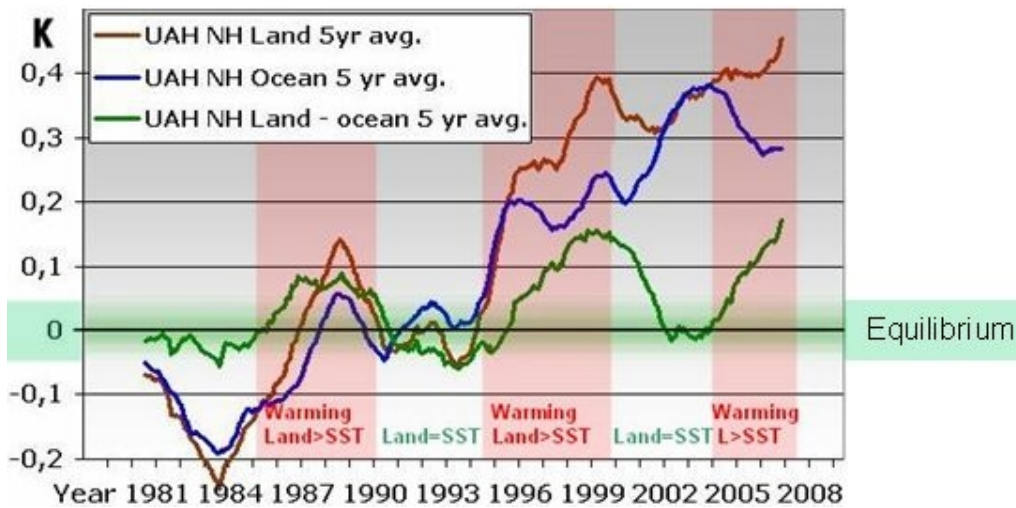
Abbildung 3: Wir wollen uns auf die zeitweiligen Lücken zwischen den Satellitendaten von Land und Wasser konzentrieren. Die grüne Kurve repräsentiert eine trendbereinigte Version, zeigt also nur den Unterschied der vom Satelliten ermittelten Temperaturwerte zwischen Land und Wasser. Aus der Abbildung 3 geht hervor, dass die Temperaturen etwa dann im Gleichgewicht sind, wenn sich die Temperatur nicht schnell ändert.
