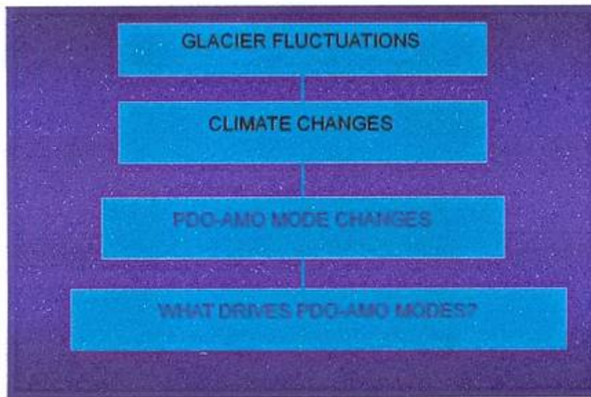
Abbildung 13: Gletschervorstöße und –rückzüge, die durch die Wassertemperatur der Ozeane beeinflusst werden. Es scheint Beweise dafür zu geben, dass die Temperatur der Ozeane durch die solare Variation beeinflusst werden, aber das muss noch näher untersucht werden.
