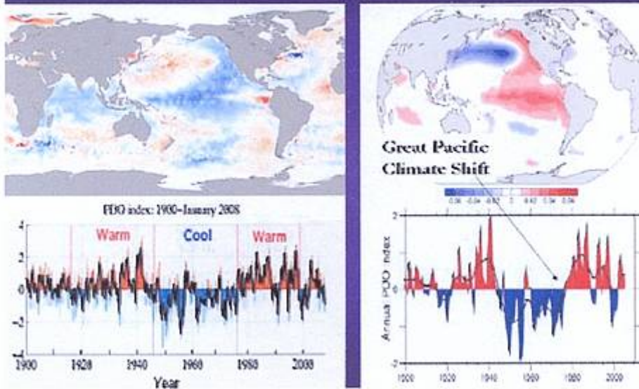
Abbildung 14: Beispiele für die Kaltphase der PDO (1945 bis 1977) und der Warmphase (1977 bis 1998).
