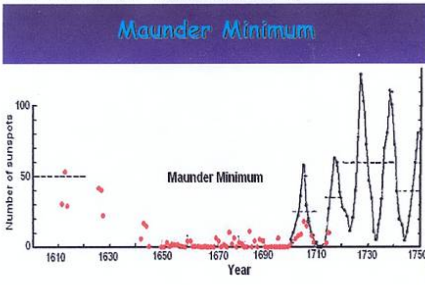
Abbildung 8: Sonnenflecken während des solaren Maunder-Minimums. Von 1650 bis 1700 wurden fast keine Sonnenflecken beobachtet, und die damit zusammenhängende Klimaabkühlung führte zu verheerenden Hungersnöten in Europa.
