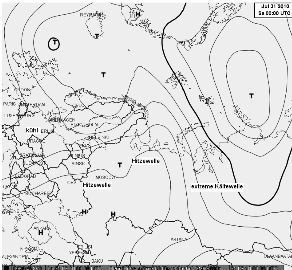
Abb. 1 Geopotential im 500-hPa-Niveau am 31.7.2010, 00 UTC Markiert ist das Gebiet, in dem die Hitzewelle auftritt. Man erkennt, dass sie am westlichen Rand eines Hochdruckkeiles im Bereich einer südlichen Strömung herrscht. Auf der Ostseite dieses Keiles reicht ein mit arktischer Kaltluft angefüllter Trog weit nach Süden, der weite Teile Mittel- und Ostsibiriens überdeckt. Dort ist es genauso zu kalt, wie es weiter westlich zu warm ist. Auch in Mitteleuropa erkennt man das mit kühler Meeresluft angefüllte Wellental. Weil aber hier die Luft vom
