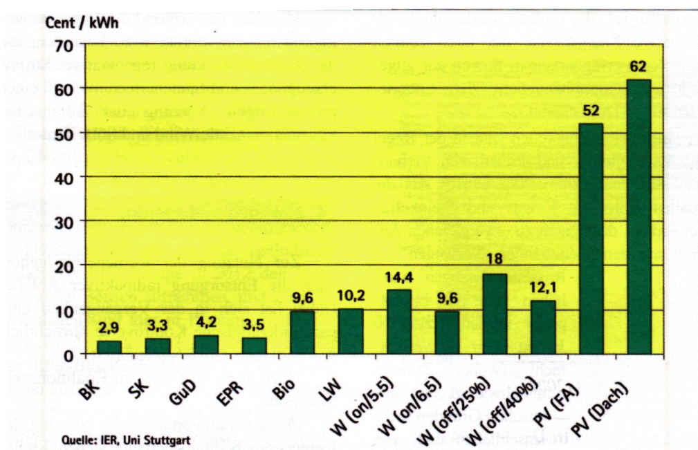
bb. 6: Stromerzeugungskosten 12 verschiedener Energiesysteme BK: Braunkohle, SK: Steinkohle, GuD: Gas- und Dampfkraftwerk, EPR TM : EPR-Reaktor, Bio: Biomasse, LW: Laufwasser, W: Wind, PV: Fotovoltaik
