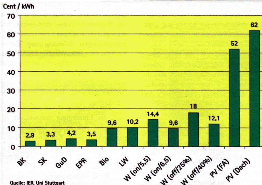
bb. 6: Stromerzeugungskosten 12 verschiedener Energiesysteme BK: Braunkohle, SK: Steinkohle, GuD: Gas- und Dampfkraftwerk, EPR TM : EPR-Reaktor, Bio: Biomasse, LW: Laufwasser, W: Wind, PV: Fotovoltaik
