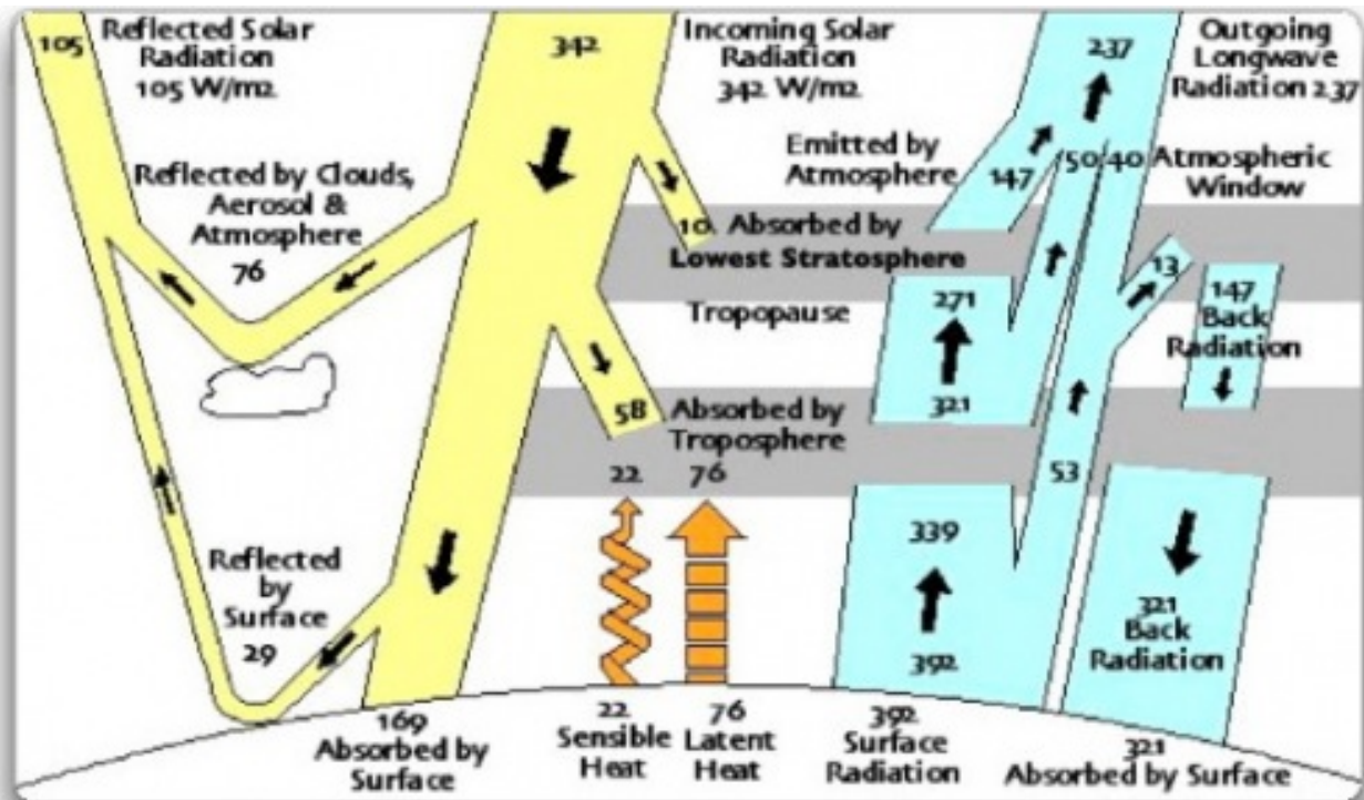
Abb. 1. Globale Energiebilanz, von Kiehl/Trenberth angepasst und erweitert. Die Werte sind Watt pro \text{qm} ( \text{W/m}^2 ). Beachte die Emission von 147 \text{ W/m}^2 am oberen Atmosphärenrand (emitted by Atmosphere). Die Tropopause ist die Höhe, wo die Temperaturabnahme mit der Höhe aufhört.
