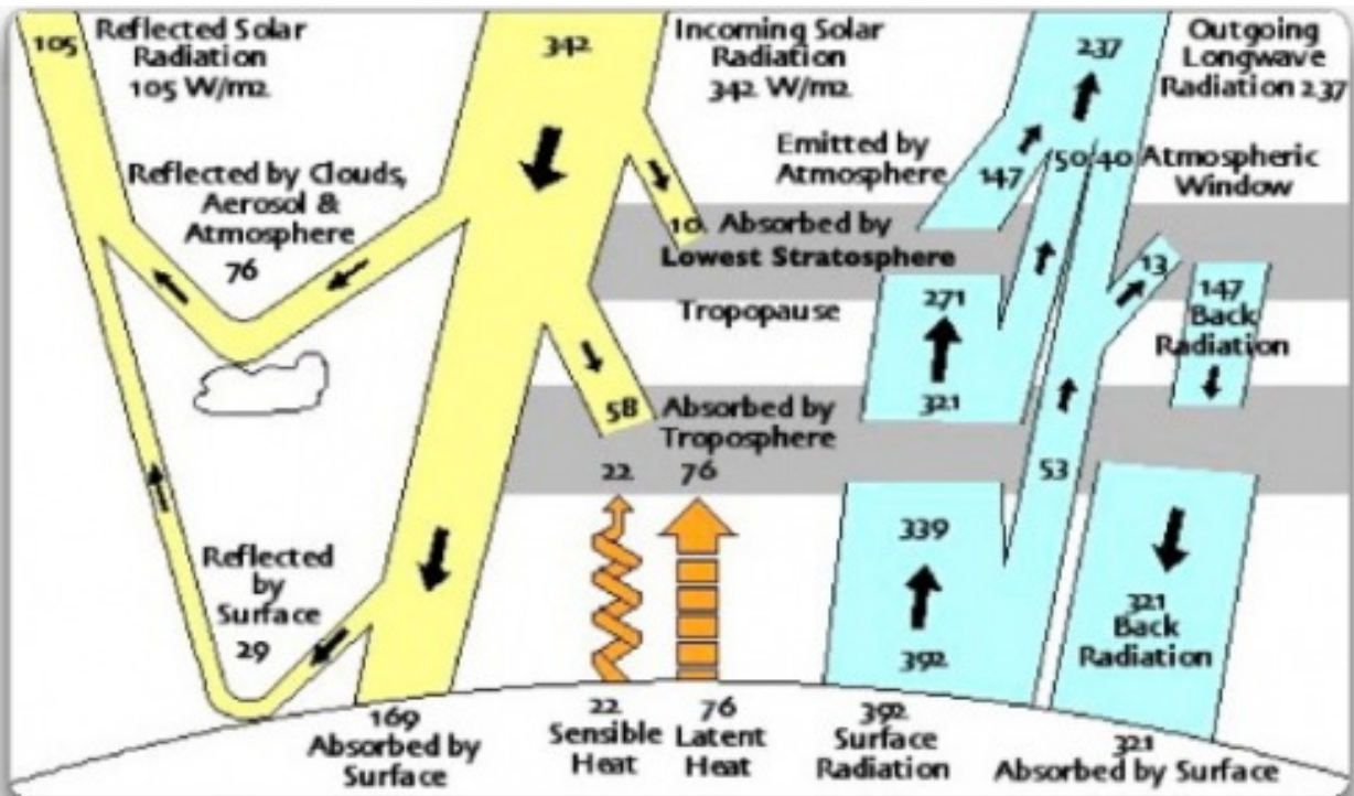
Abb. 1. Globale Energiebilanz, von Kiehl/Trenberth angepasst und erweitert. Die Werte sind Watt pro qm (W/m 2 ). Beachte die Emission von 147 W/m 2 am oberen Atmosphärenrand (emitted by Atmosphere). Die Tropopause ist die Höhe, wo die Temperaturabnahme mit der Höhe aufhört.
