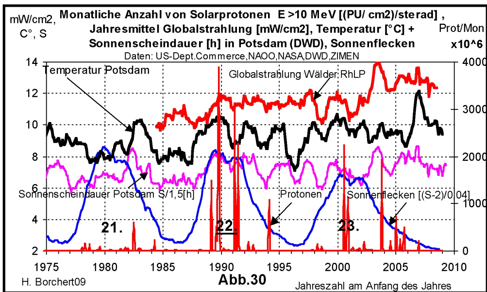
Abb. 30: Globalstrahlung, Sonnenscheindauer und Sonnenaktivitat
