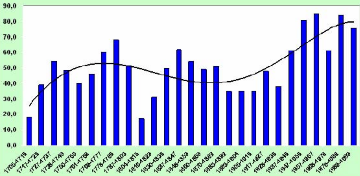
Abb. 6 Mittlere Sonnenfleckenzahl je Sonnenfleckenzyklus 1705 - 1999
