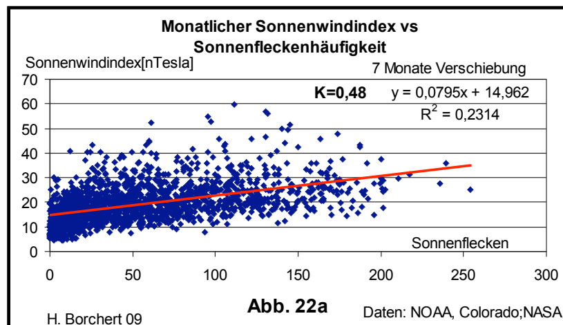
Abb. 22a: Korrelation des monatlichen Sonnenwindindex Sonnenfleckenhäufigkeit
