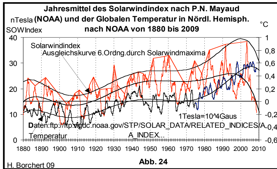
Abb.24: Vergleich des Verlaufs der Maximalwerte des SOWI-Index mit Temperaturverlauf
