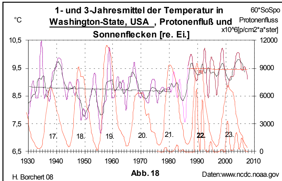
Abb. 18: Temperaturverlauf in Bundesstaat Washington und solarer Protonenstrom
