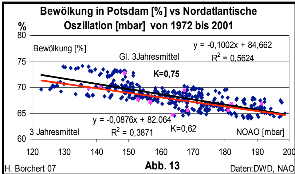
Abb.13: Bewölkung in Potsdam vs Nordatlantische Oszillation
