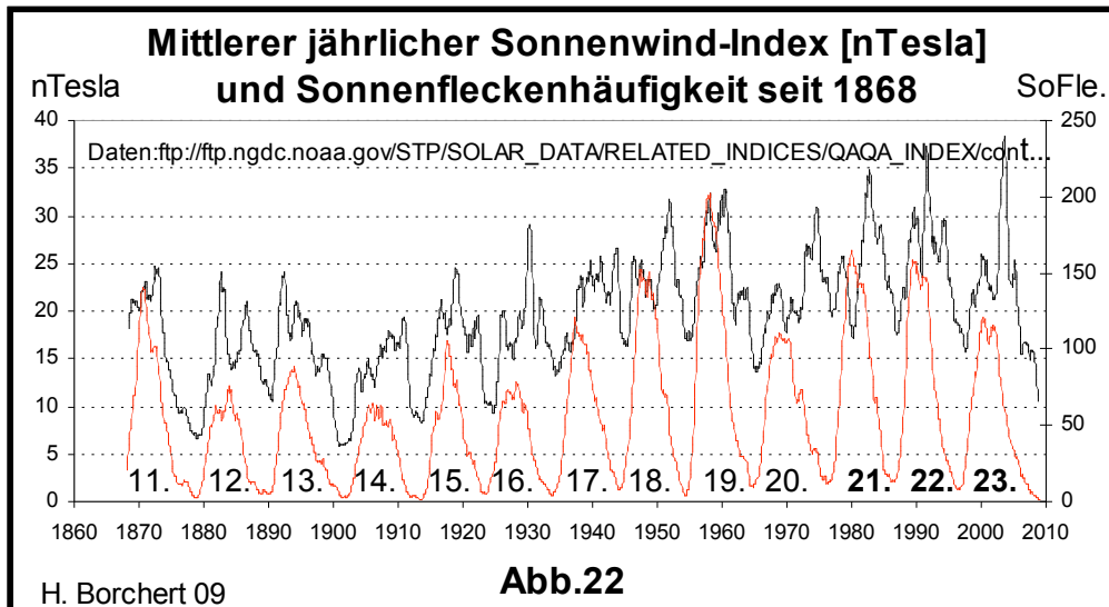
Abb.22: Mittlerer jährlicher Sonnenwind-Index und Sonnenfleckenhäufigkeit
