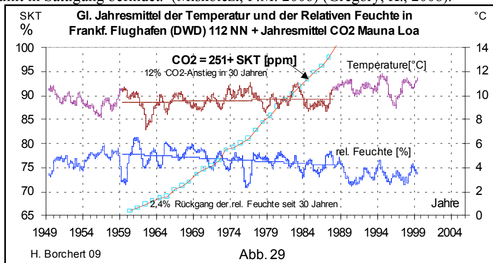
Abb.29. Rückläufige relative Feuchte bei ansteigender CO 2 -Konzentration
