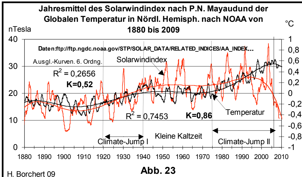
Abb.23: Sonnenwind-Index und Verlauf der Globaltemperatur nach NOAA seit 1880
