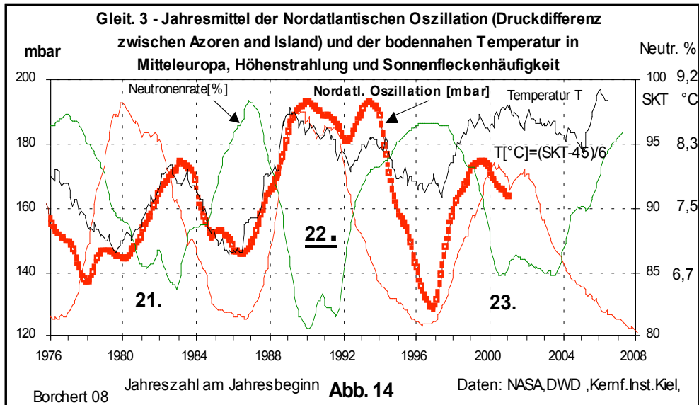
Abb.14 : Nordatlantische Oszillation, Höhenstrahlung und Temperatur in Deutschland
