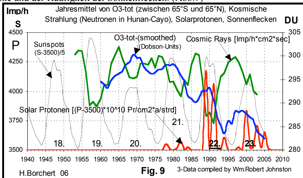
Abb. 9: Abbau stratosphärischen Ozons durch Kosmische Strahlung und Protonen
