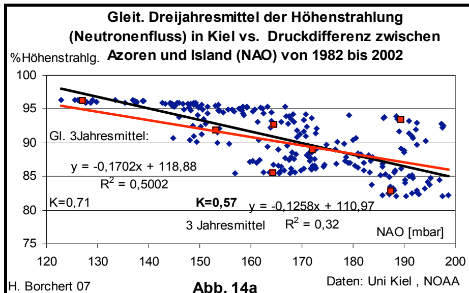
Abb.14a.: Nordatlantische Oszillation korreliert mit der Höhenstrahlung
